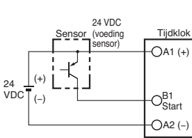
Werkt wanneer de PNP-transistor inschakelt.
