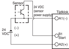
Werkt wanneer de NPN-transistor inschakelt.
