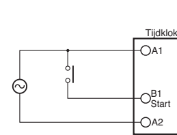
Werkt wanneer het relais inschakelt.
